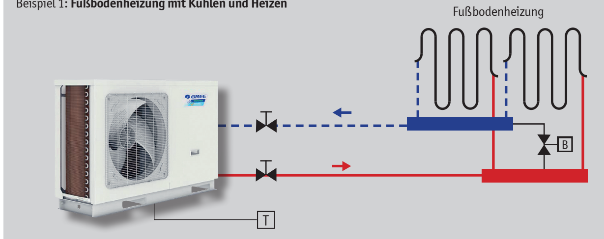
Beispiel 1: Fußbodenheizung mit Kühlen und Heizen
