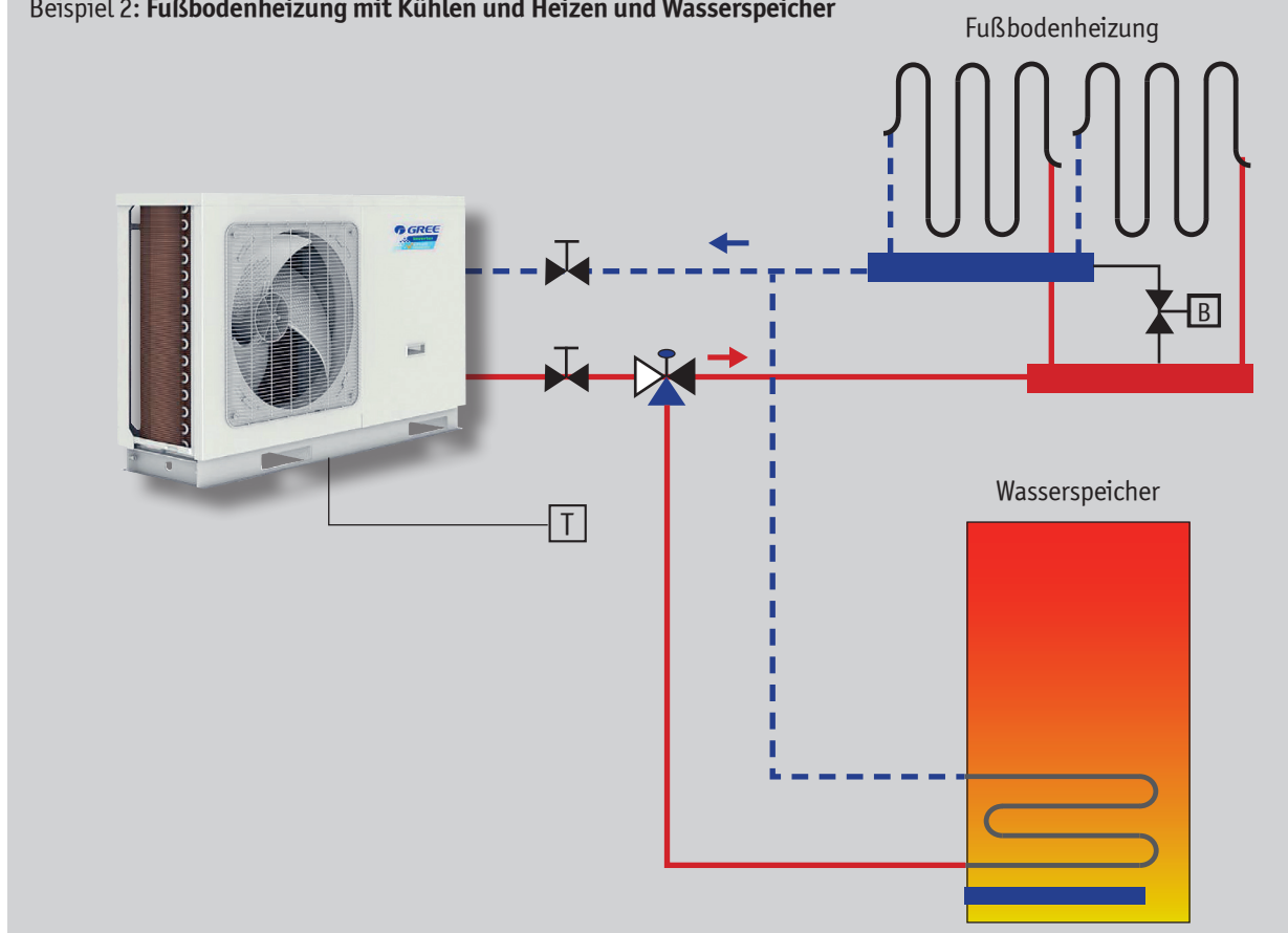
Beispiel 2: Fußbodenheizung mit Kühlen und Heizen und Wasserspeicher
