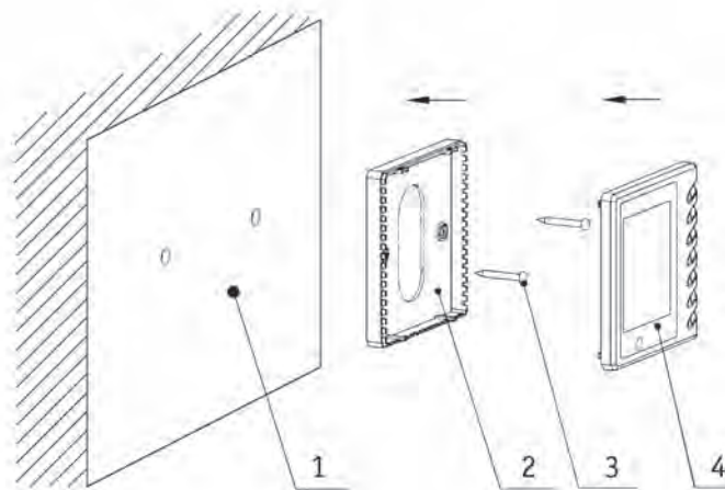
Installationsschema
