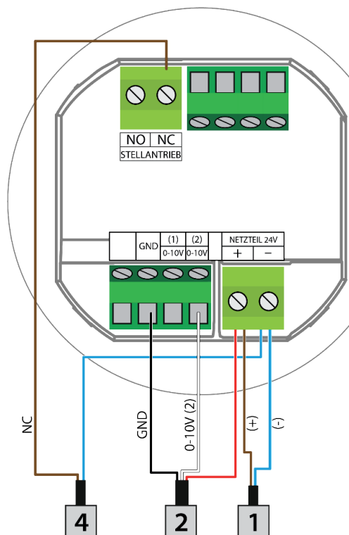
3. Anschluss des NC-Stellantriebs
